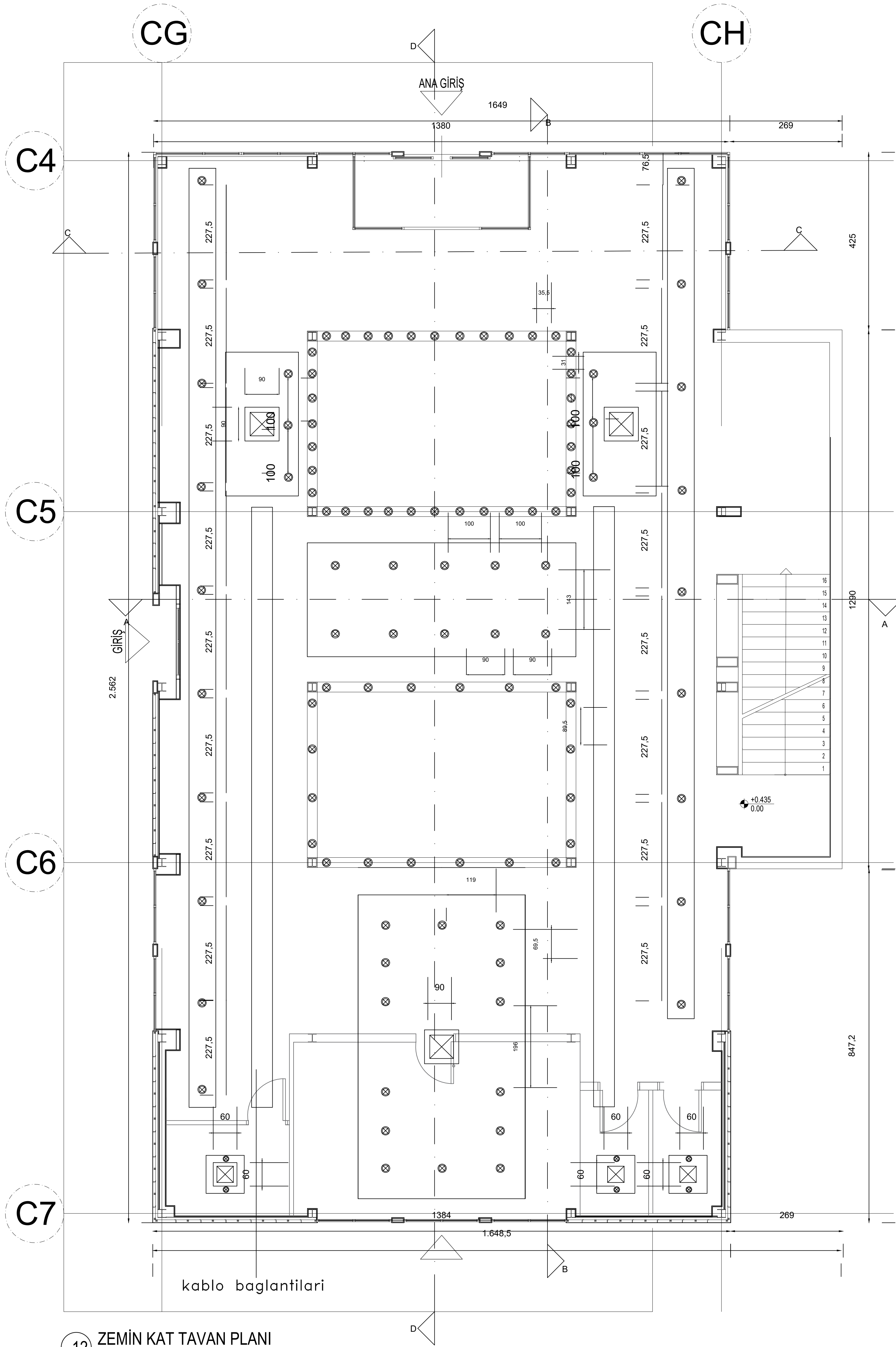
12 ZEMİN KAT TAVAN PLANI ÖLÇEK:1/50
