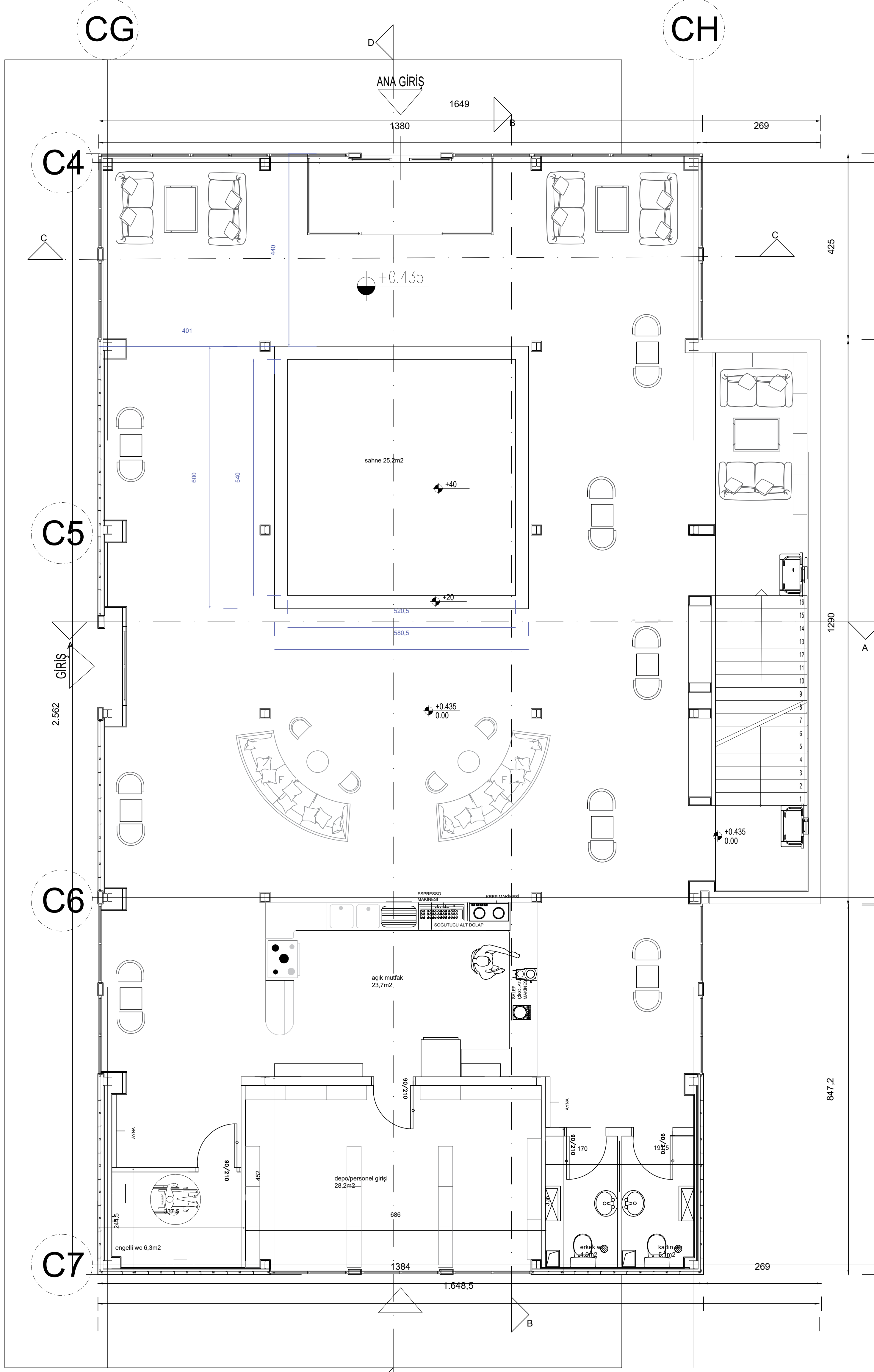
3 ZEMİN KAT PLANI ÖLÇEK:1/50
