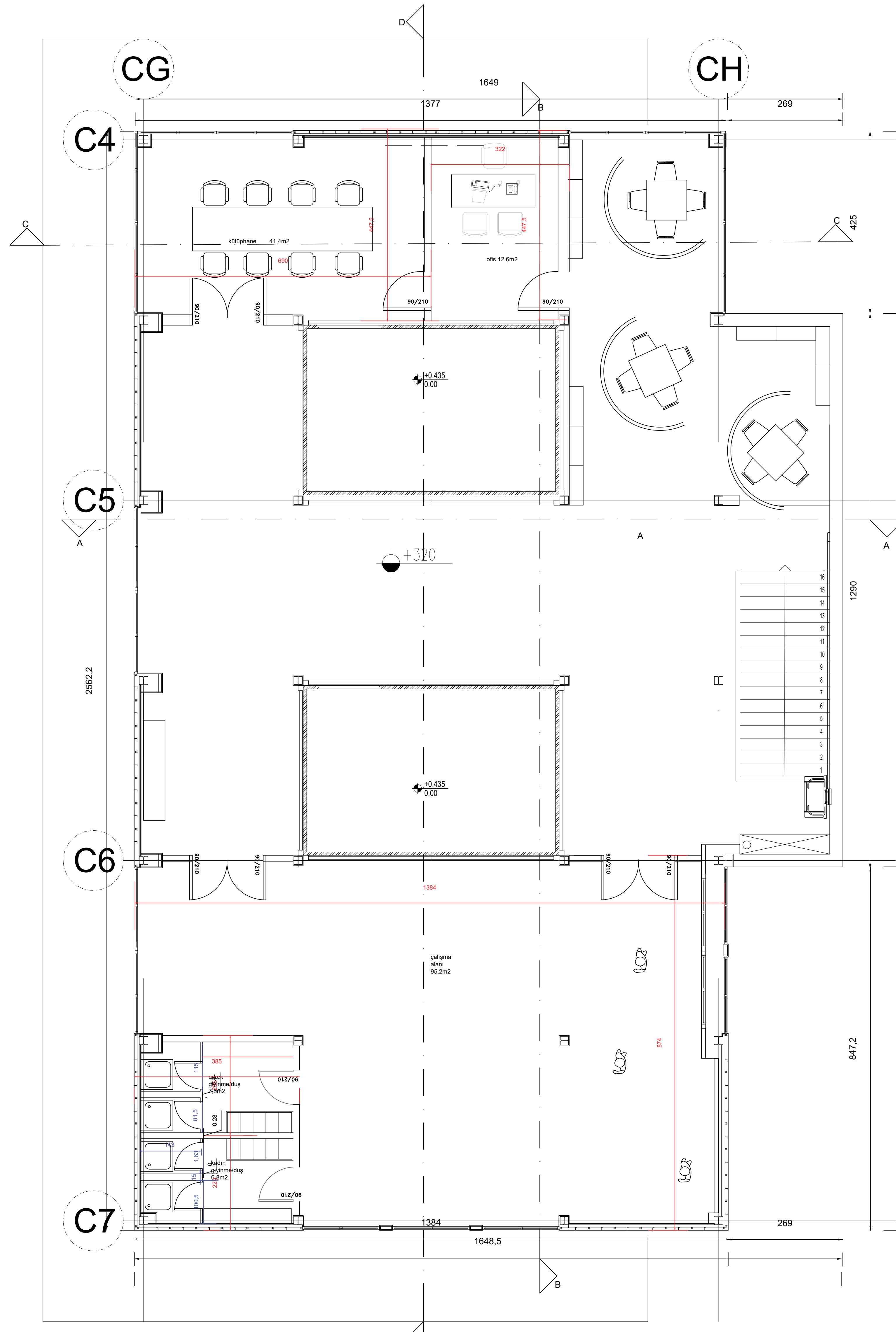
4 GALERİ KAT PLANI ÖLÇEK:1/50
